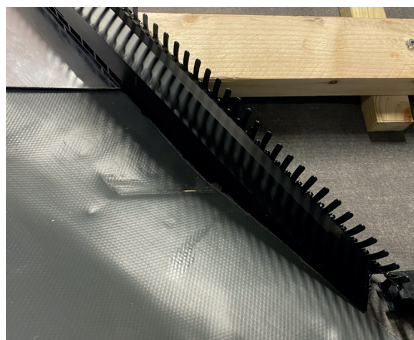
4. Afslut med et helt element som tildannes, så det passer til hældning på tagfod.
