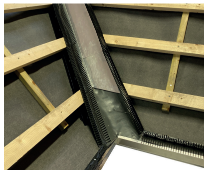
6. Skotrende med færdigmonterede skotrende elementer. Klar til oplægning af tagsten.
