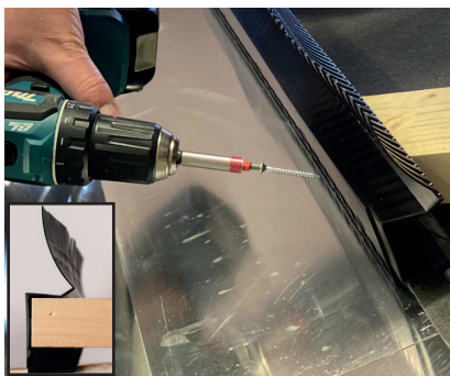
2. Fastgør med skrue i lægten fra siden eller fra oven.
