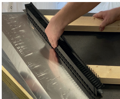
1. Klem første skotrende element fast omkring tilstødende lægte.
