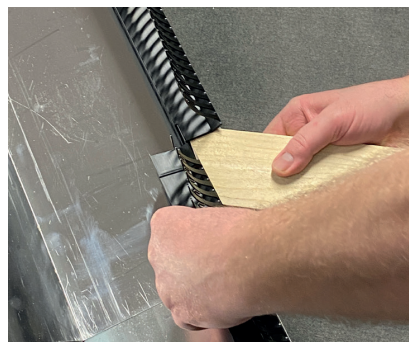
3. Klik næste element på og fastgør på samme måde.
